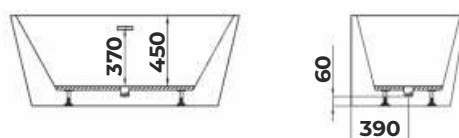
SEKCJA A-A
