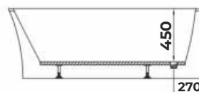
SEKCJA A-A
