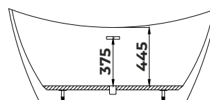
SEKCJA A-A
