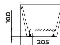
SEKCJA B-B
